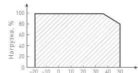
Рис. 2. Максимальная допустимая нагрузка, % от мощности источника
