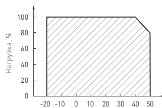
Рис. 3. Максимальная допустимая нагрузка, % от мощности источника
