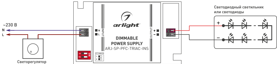
Рисунок 1. Подключение источника питания при использовании интерфейса TRIAC
