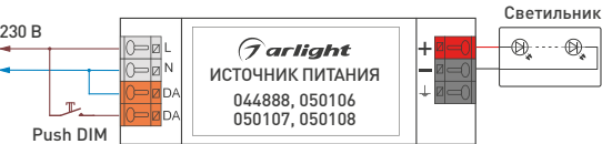
Рис. 3. Подключения источника питания с управлением Push DIM
