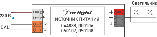
Рис. 2. Подключения источника питания с управлением DALI
