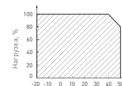
Рис. 3. Максимальная допустимая нагрузка, % от мощности источника
