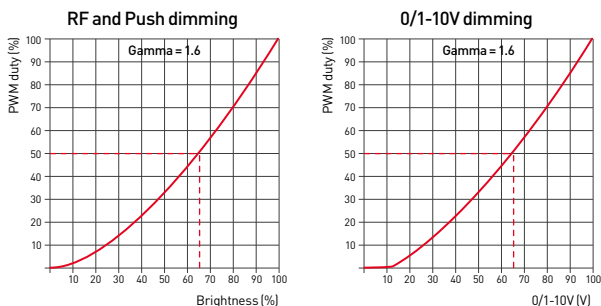
Рис. 2. Кривые диммирования в зависимости от типа управления
