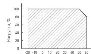
Температура окружающей среды (t amb ), °C Рис. 3. Максимальная допустимая нагрузка, % от мощности источника
