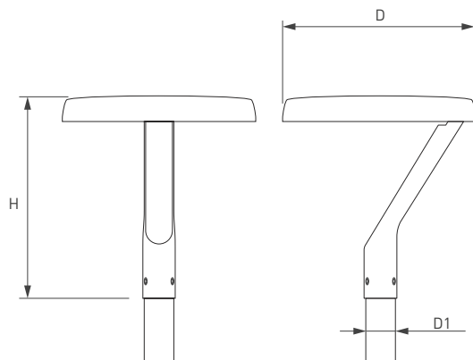
Рис. 1. Чертеж и габаритные размеры
